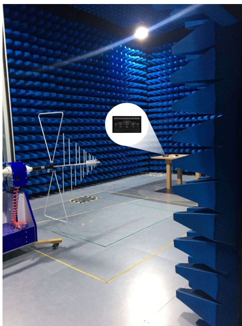
图 5-4 RE 测试图
