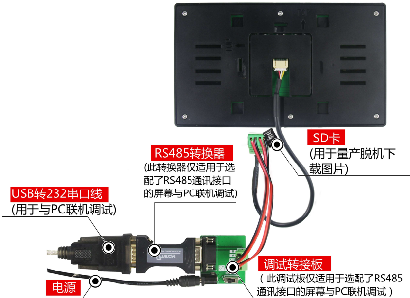
图 1-4 调试工具图
