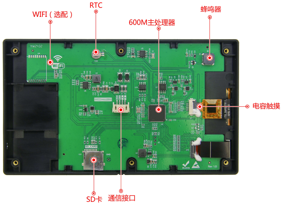
图 1-3 硬件配置图
