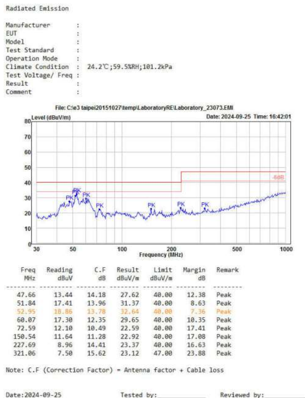
图 5-6 RE 测试垂直方向
